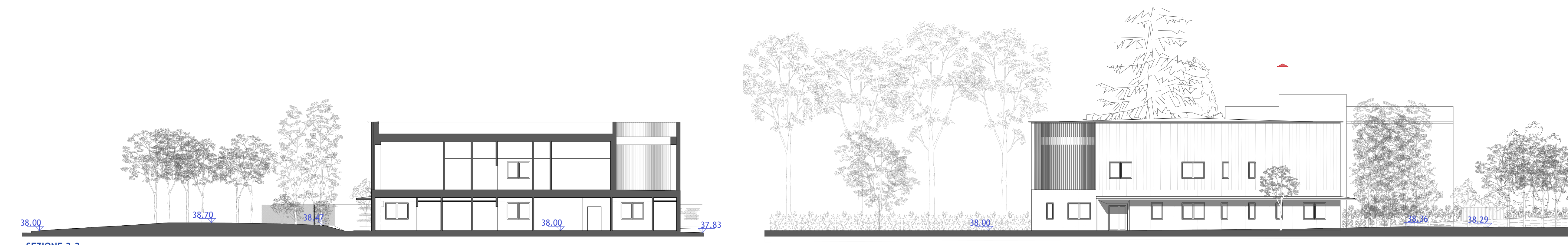
SEZIONE 3-3
